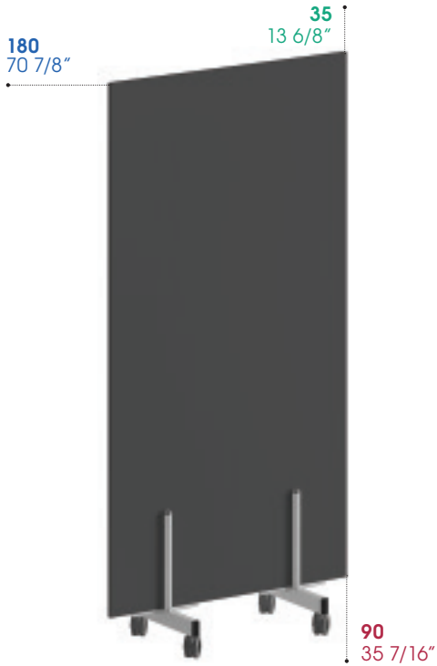
Partizione in melaminico sp. 1,8 cm con base su ruote / Melamine partitions 3/8" thick, with base on castors
